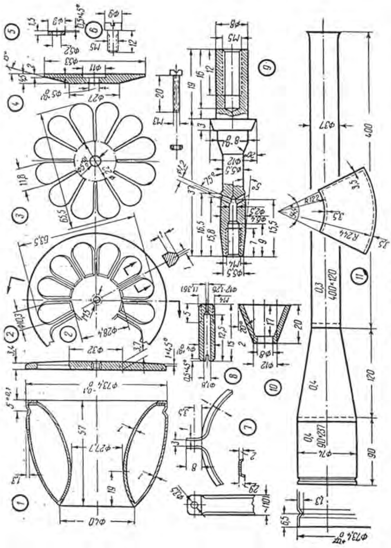
Рис. 63. ПуВРД Аэроджет-2:
